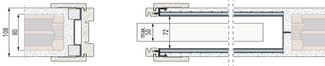
Dokončená tloušťka stěny 125 mm - hrubá tloušťka 100 mm
