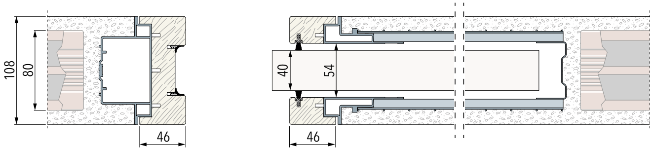
Dokončená tloušťka stěny 125 mm - hrubá tloušťka 100 mm
