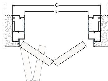
SKLÁDACÍ NÁBYTKOVÉ DVEŘE
