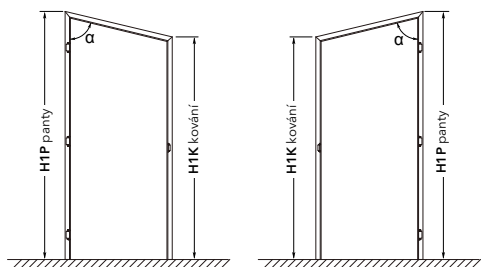
ZÁRUBEŇ S VRCHNÍM PROFILEM
