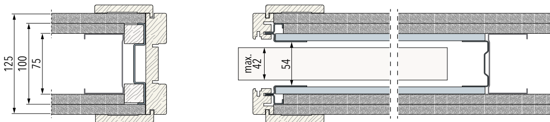
Dokončená tloušťka stěny 125 mm: pouzdro 125 mm - pro profil 75 mm - 1x opláštění pouzdra, 2x opláštění SDK příčky.
