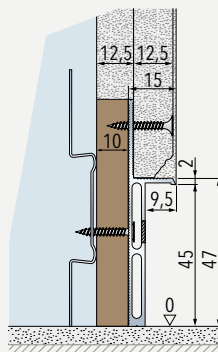
Soklový profil 15 mm na SDK stěně při dvojitém opláštění
