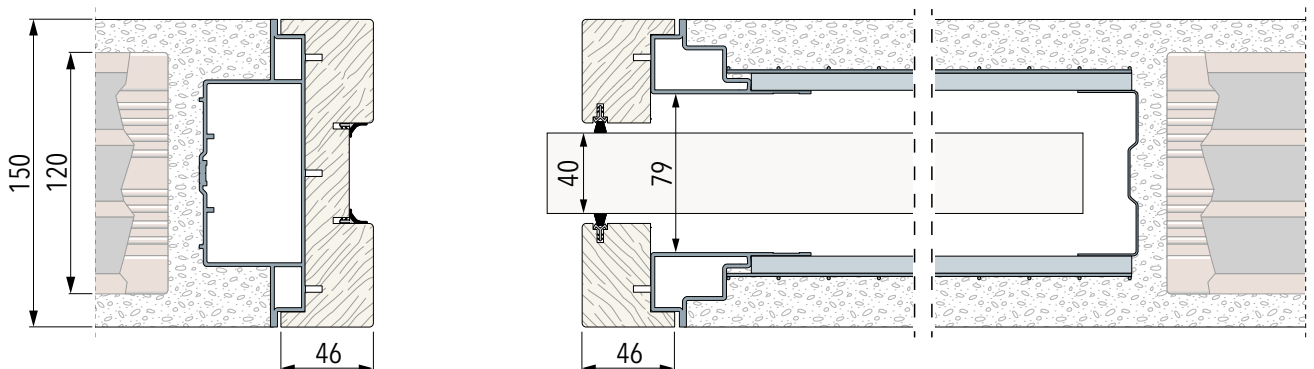
Dokončená tloušťka stěny 150 mm - hrubá tloušťka 120 mm
