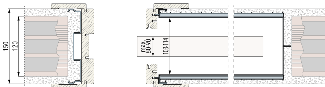
Dokončená tloušťka stěny 150 mm - hrubá tloušťka 120 mm
