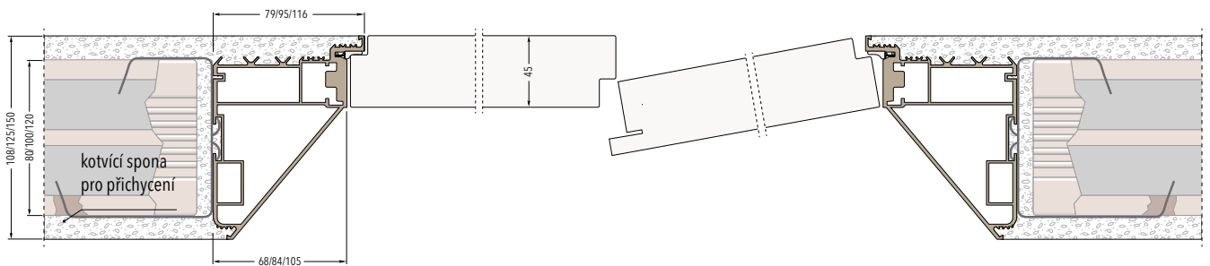
PRAVÉ DVEŘE OTEVÍRANÉ DOVNITŘ - LEVÉ FIX
