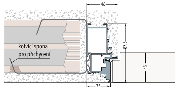
TÁHNOUT (otevřít dovnitř; k sobě)
