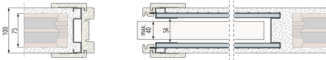
Dokončená tloušťka stěny 100 mm - hrubá tloušťka 75 mm
