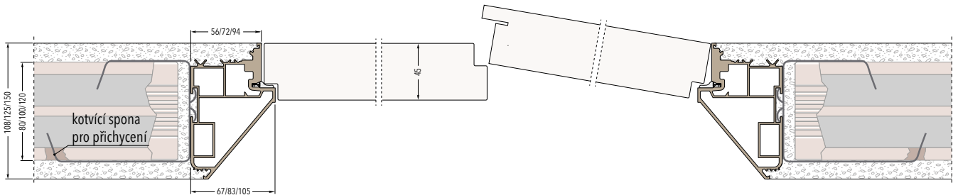
PRAVÉ DVEŘE OTEVÍRANÉ VEN - LEVÉ FIX
