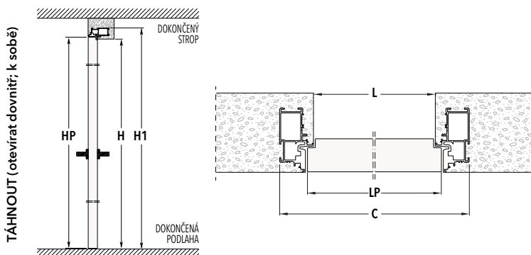
ZÁRUBEŇ S VRCHNÍM PROFILEM
