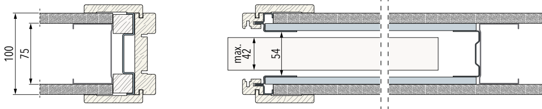
Dokončená tloušťka stěny 125 mm: pouzdro 100 mm - pro profil 75 mm - 2x opláštění SDK. Obložka na 100 mm
