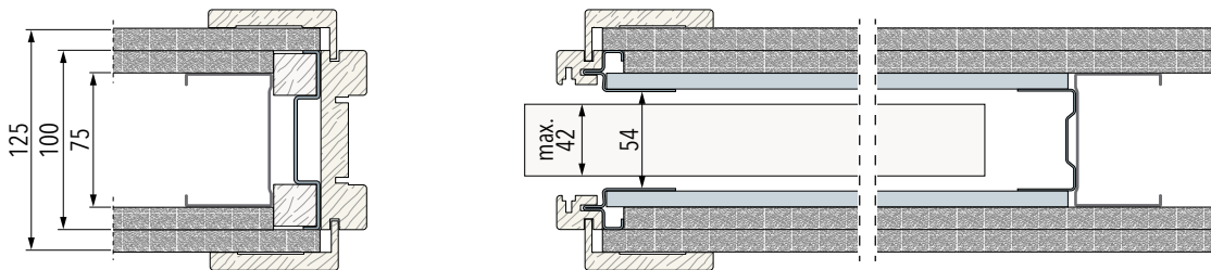
Dokončená tloušťka stěny 125 mm: pouzdro 125 mm - pro profil 75 mm - 2x opláštění SDK. Obložka na 125 mm
