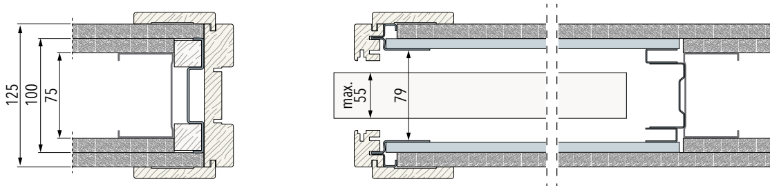
Dokončená tloušťka stěny 125 mm: pouzdro 125 mm - pro profil 100 mm - 1x opláštění SDK
