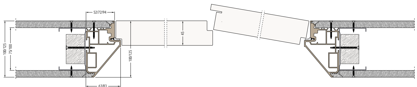
PRAVÉ DVEŘE OTEVÍRANÉ DOVNITŘ - LEVÉ FIX
