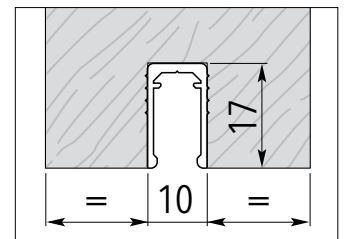
Detail vsunutého ochranného profilu
